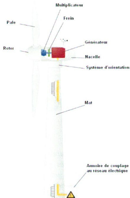
Schéma d'une éolienne
